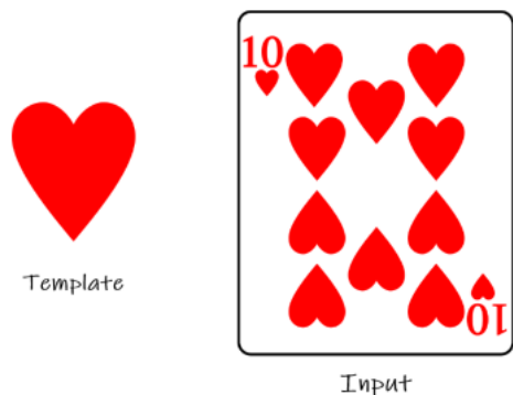
Figura 21: Valores de entrada para Multi-Template Matching [32]
