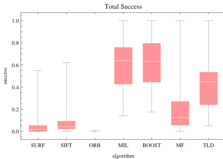
Figura 23: Taxa de sucesso dos algoritmos de rastreamento do OpenCV [30]
