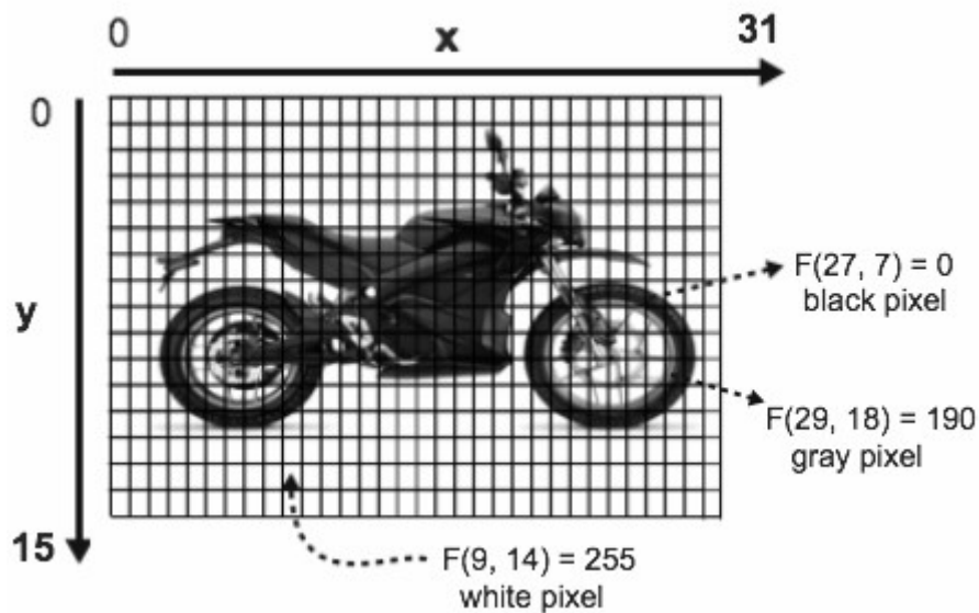
Figura 3: Matriz de uma imagem em tons de cinza [20]
