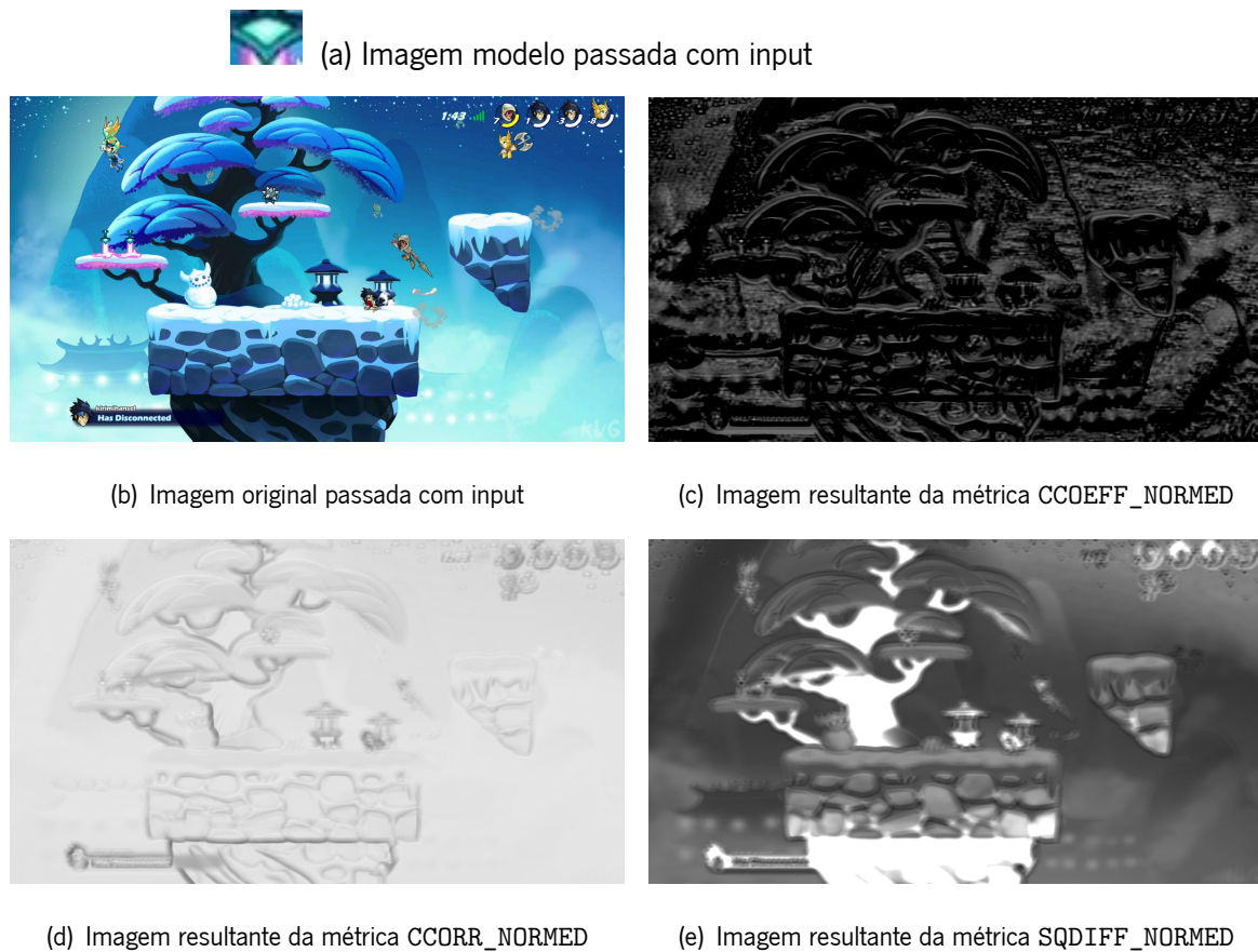
Figura 31: Imagens de input e output da função matchTemplate() com as diferentes métricas normalizadas possíveis
