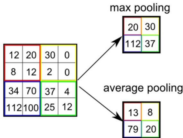
Figura 7: Tipos de Pooling [54]
