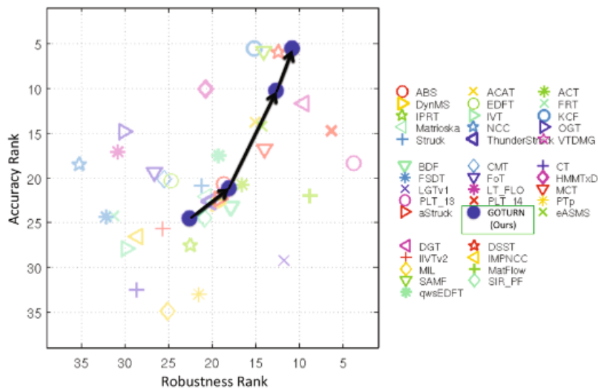
Figura 25: Comparação dos vários algoritmos de rastreamento relativamente a exatidão e robustez [28]
