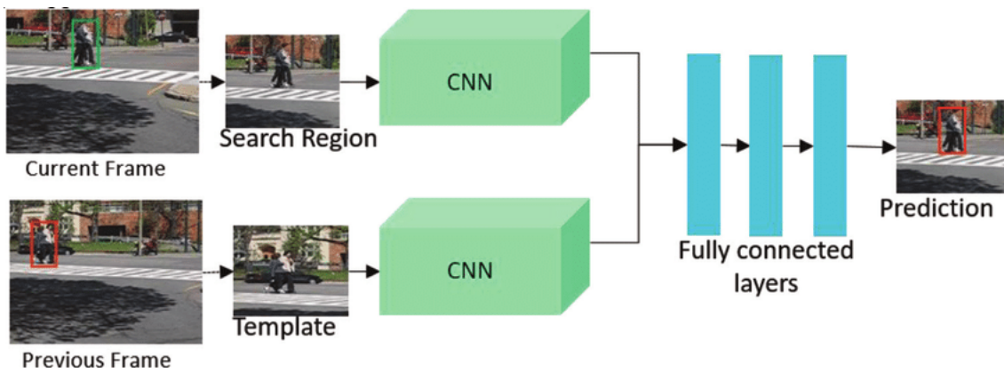
Figura 33: Arquitetura do rastreamento do algoritmo GOTURN
