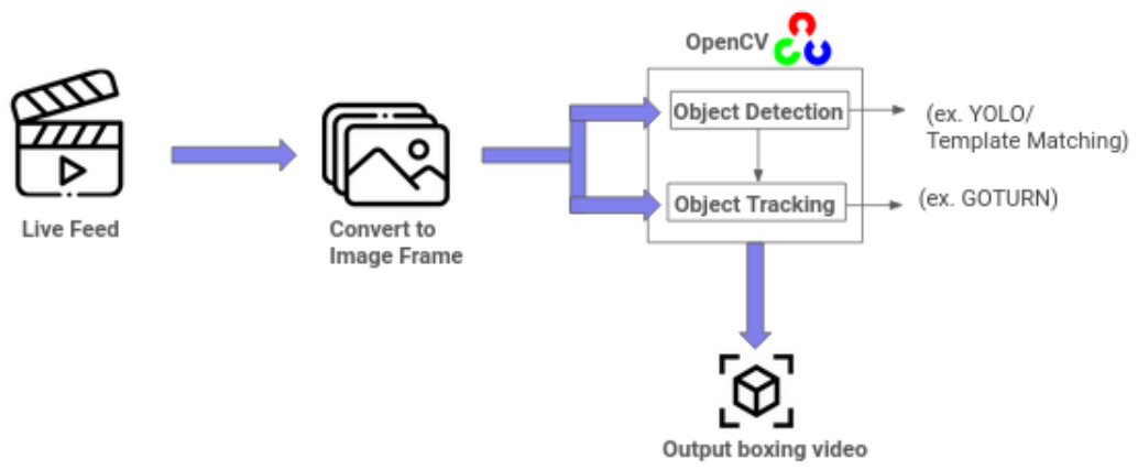
Figura 26: Fluxo de dados
