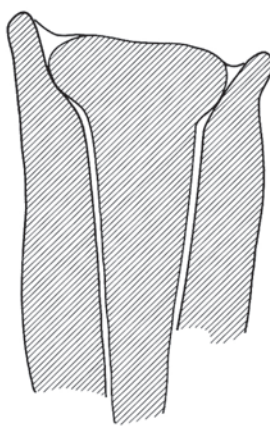
Figura 4. a – Cone de vazamento com os jitos (perfurações) correspondendo ao alvado da ponta de lança (Ref. 2006-0139); b – Desenho do que resta do molde de cera perdida de uma ponta de lança de alvado (Ref. 2006-0139).
