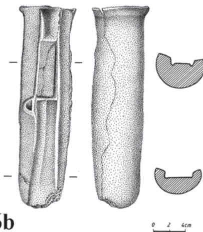
Figura 6. a – Parte de molde bivalve cerâmico de machado de talão conservando o talão e parte do gume com, pelo menos, uma argola (identificável ao centro do lado esquerdo) e o cone de vazamento no topo (Ref. 2006-0338); b – Desenho de parte do gume do molde bivalve cerâmico de machado de talão com pelo menos uma argola.
