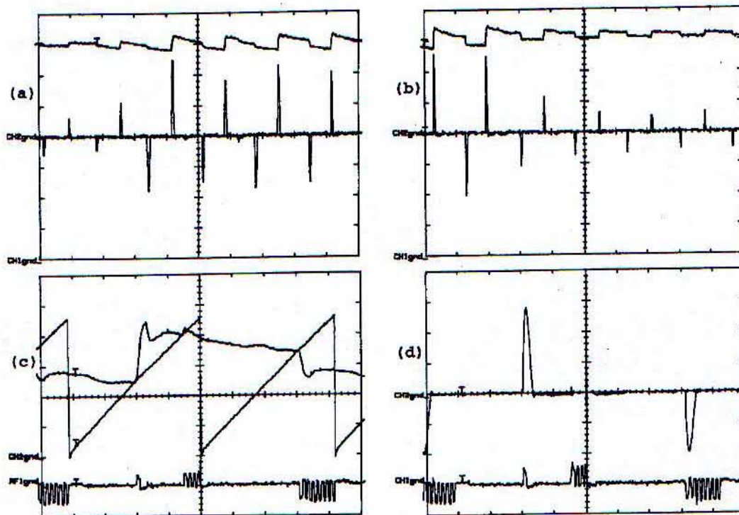
Figura 3 - Tensão de saída e corrente de entrada no rectificador em cascata de 10 KV para operação com o regulador a tirístores: (a) quando do aumento da carga, (b) quando da redução da carga. (c) Tensão dente de serra e tensão de referência para o TCA 780, e pulsos de disparo. (d) Corrente de entrada do rectificador em cascata e pulsos de disparo.
