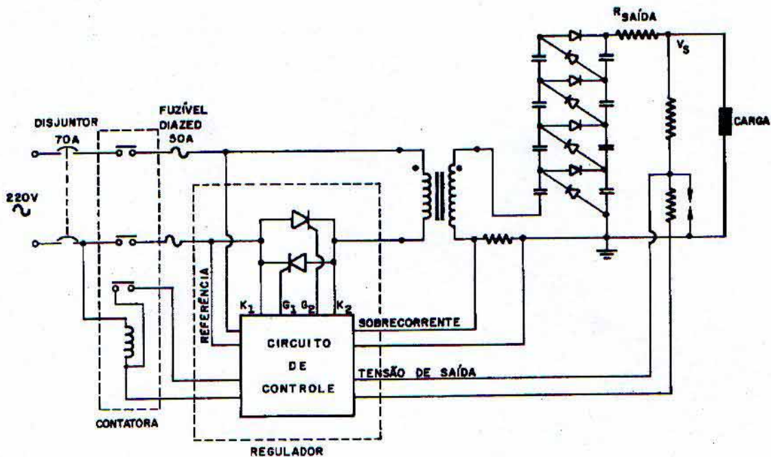
Figura 1 - Circuito do rectificador em cascata com regulador a tirístores.
