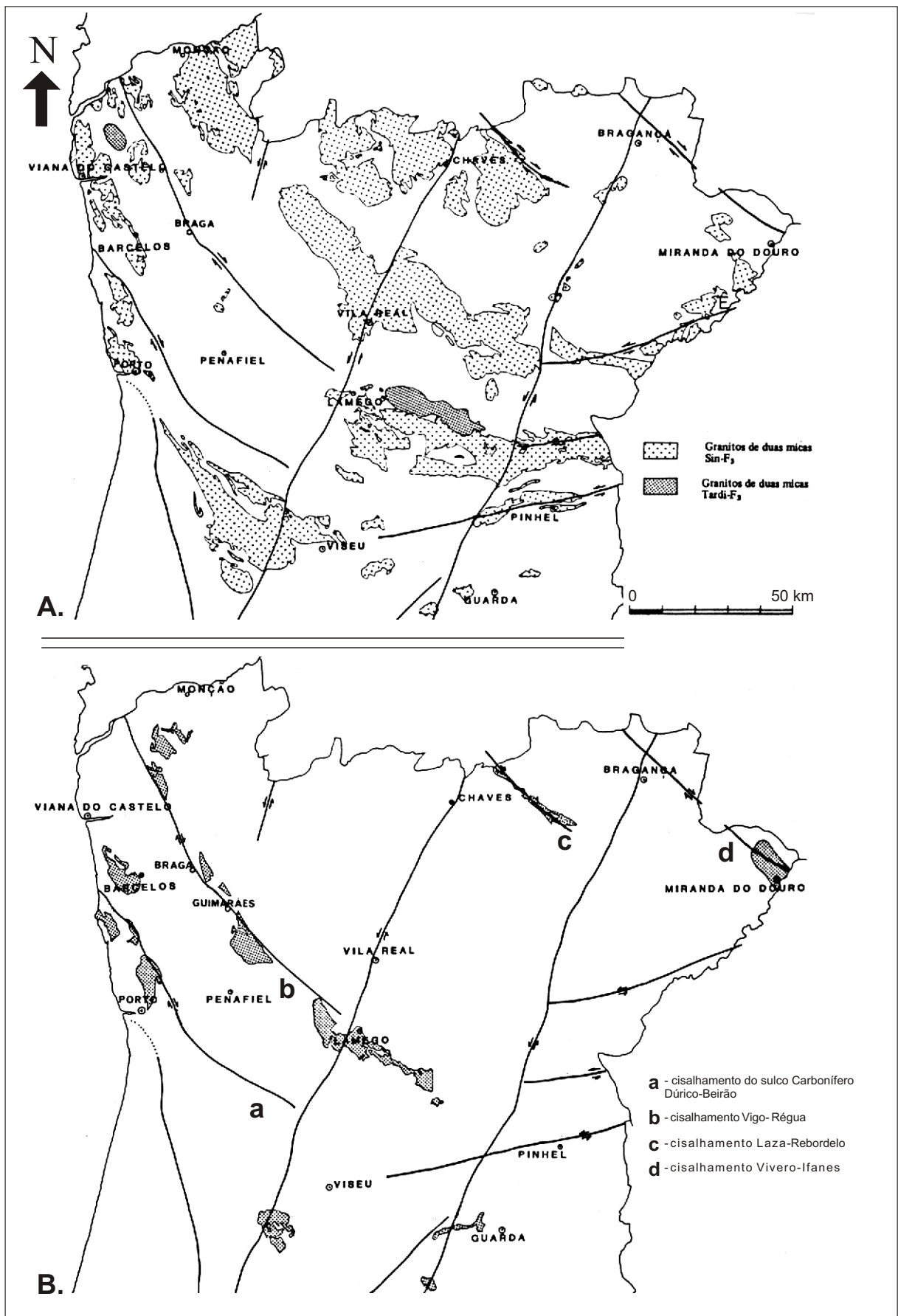
Figura.II.18- Distribuição de granitóides sinorogénicos. A. granitóides de duas micas (sin-F 3 e tardi-F 3 ); B. granitóides biotíticos sin-F 3 . Adaptado de Ferreira et al. (1987).
