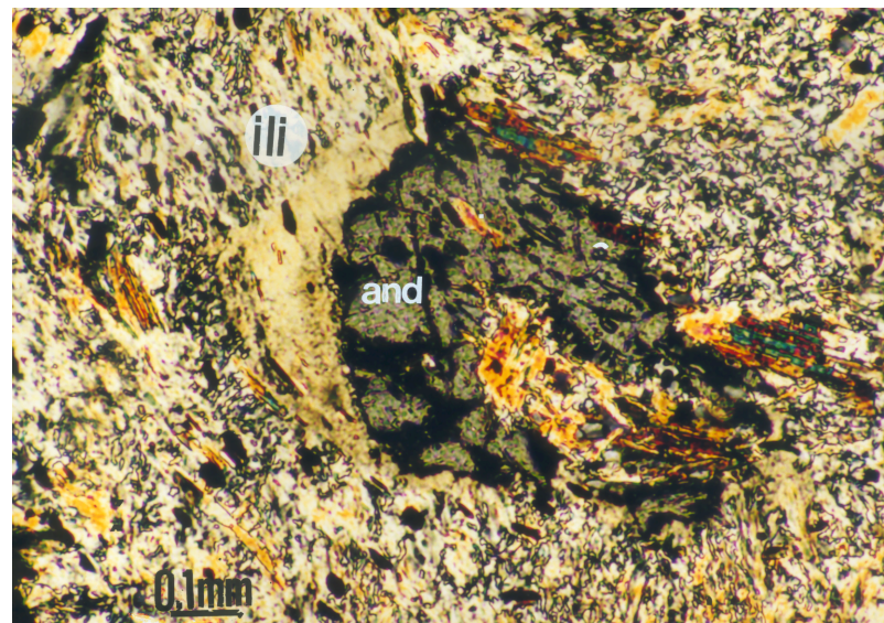
Figura2- Micaxisto com nódulos de andaluzite. Relíquia de andaluzite (and) numa massa de alteração de ilites (ili). M-O. (nicóis cruzados).
