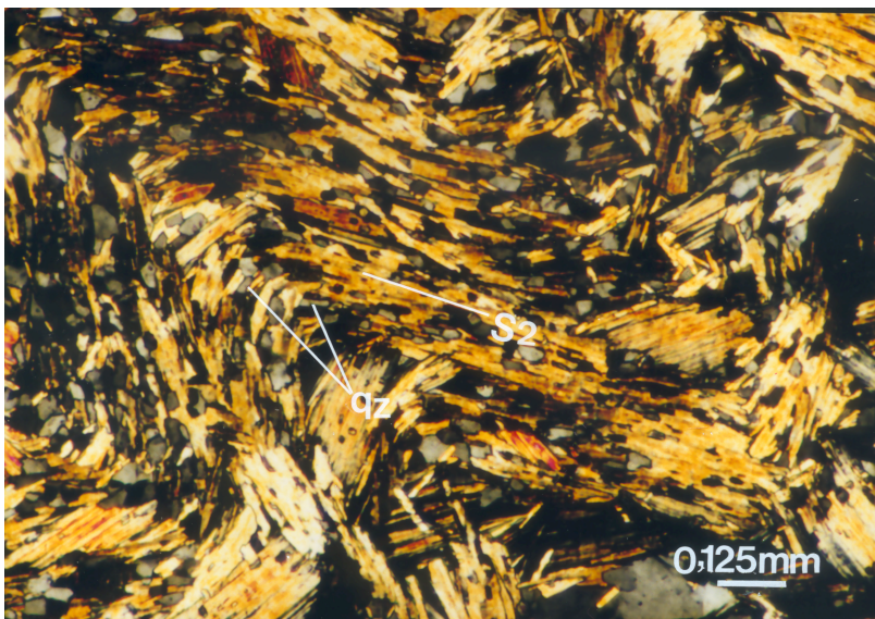
Figura1- Micaxisto evidenciando crenulação da superfície S 2 . Na nota-se a presença de quartzo (qz) deformado. M-O. (nicóis cruzados).
