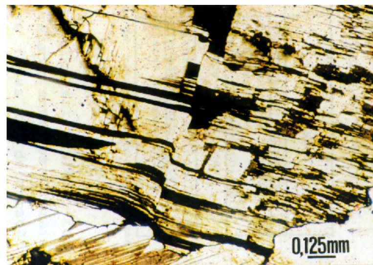
Figura4- Aplito-pegmatito com plagioclase (albite) deformada em dúctil e dúctil-frágil. M-O. (nicóis cruzados).
