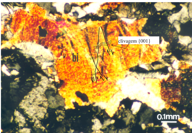
Figura3- Secção de biotite (bi), pertencente a uma conjunção de kinks (nicóis cruzados).
