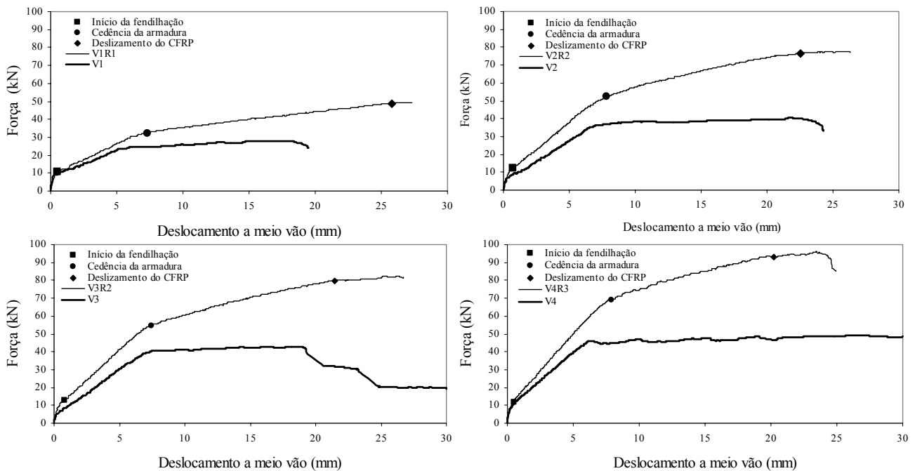
Figura 10 - Diagramas carga vs flecha das vigas.
