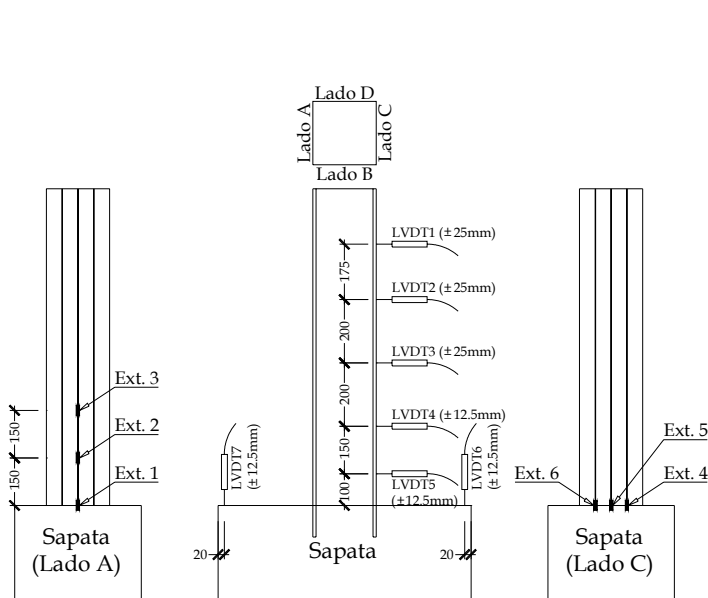
Figura 3 - Localização dos transdutores de deslocamentos, LVDT's, e dos extensómetros, ext (dimensões em milímetros).
