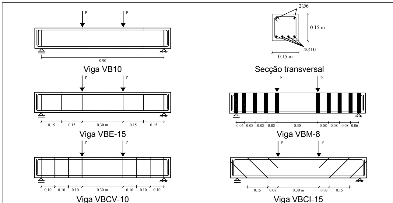
Figura 12 - Modelos VB10, VBE-15, VBM-8, VBCV-10 e VBCI-15.
