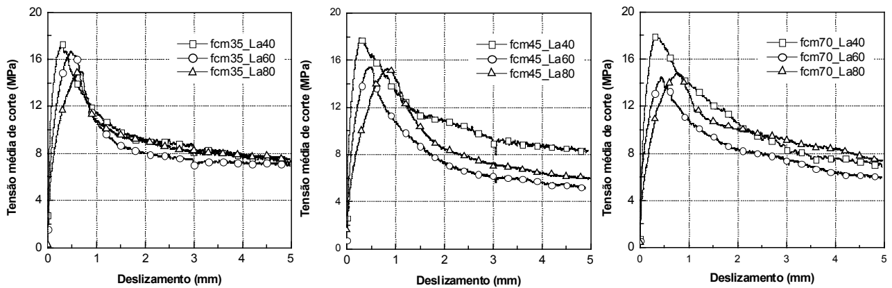
Figura 17 - Influência de fcm na relação tensão média de corte vs deslizamento.
